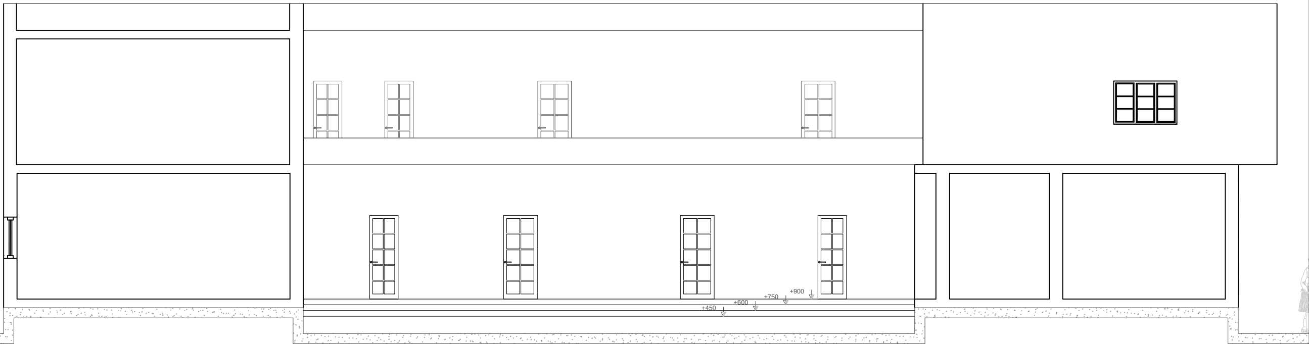
SECTION A-A'
